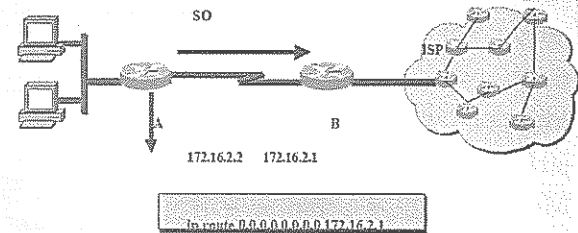
Gambar 3. Paket yang dikirim melalui default gateway router B
