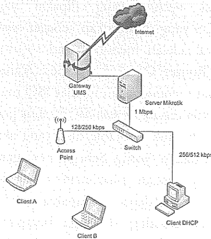
Gambar 5. Konfigurasi jaringan komputer yang dipakai penelitian untuk client dinamis
