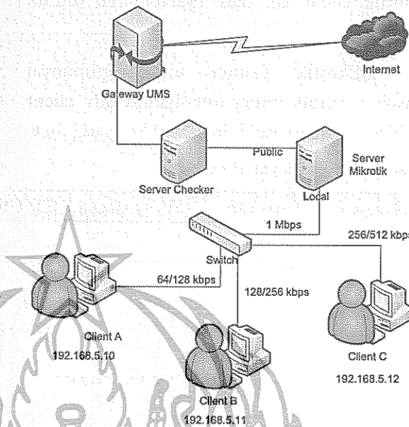
Gambar 7. Susunan jaringan computer dalam pengujian di FT. UMS
