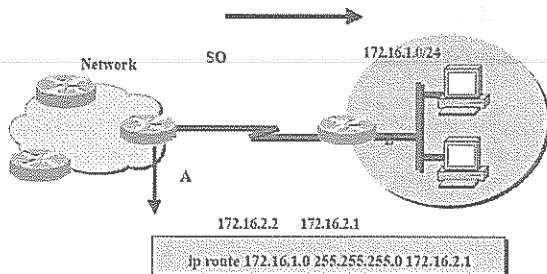
Gambar 2. Terapan static router B sebagai gateway
